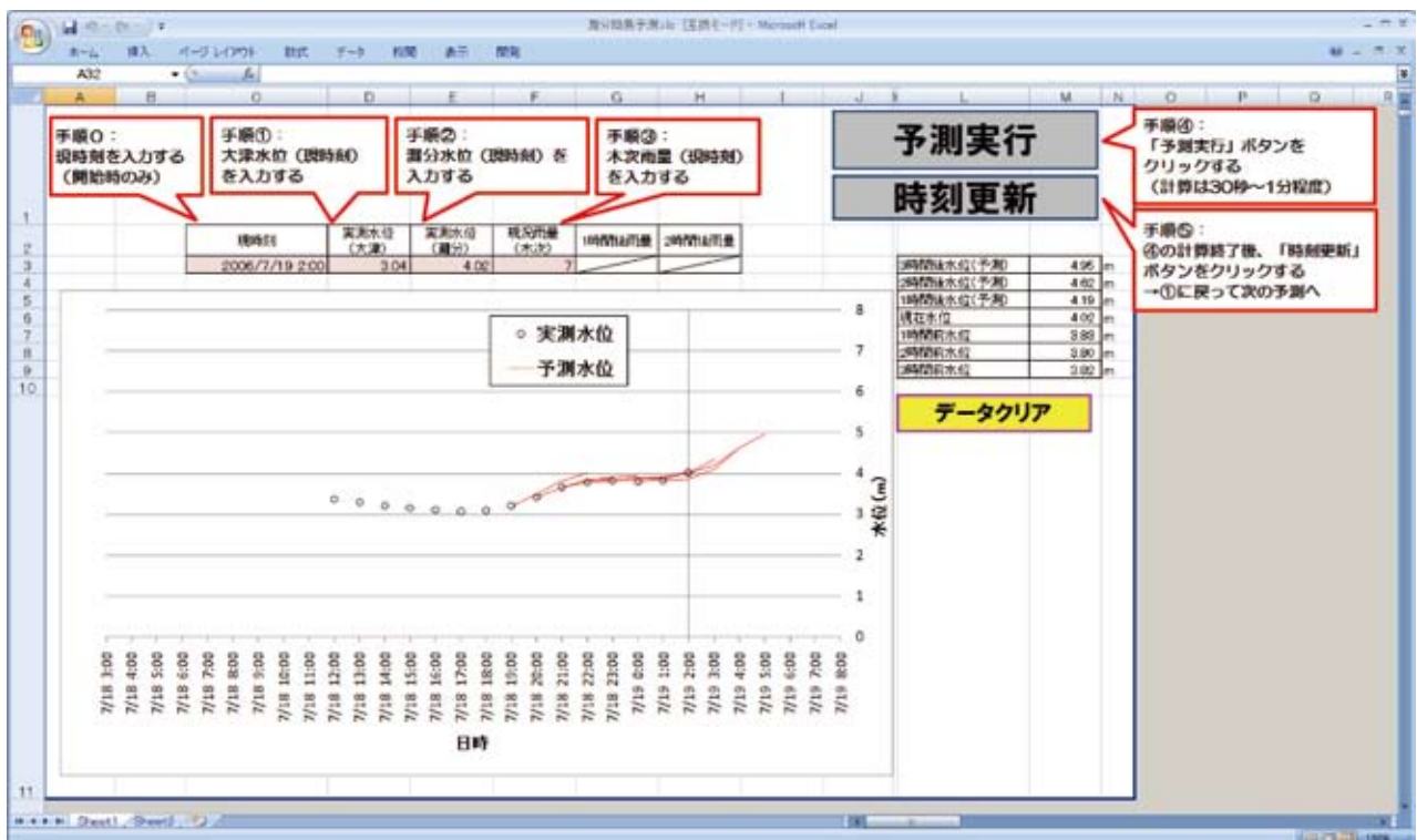
図－10 予測システムの表示画面例
