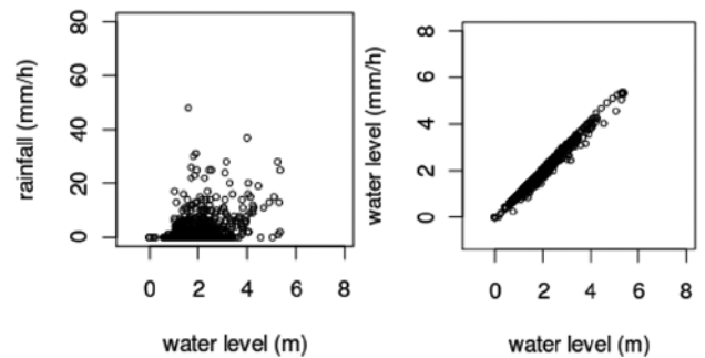
図－5 相関分布（左：水位－雨量、右：水位－水位）
