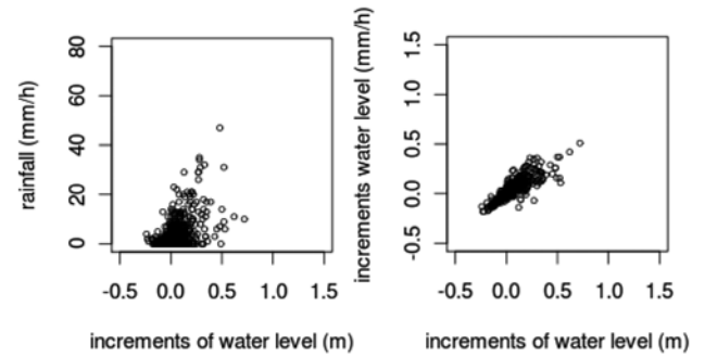
図－4 相関分布（左：水位変化－雨量、右：水位変化－水位変化）
