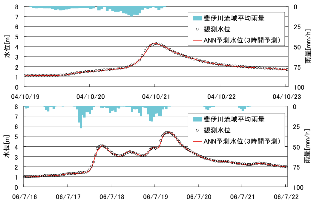
図-8 灘分地点における洪水予測の検証結果 (04年10月、06年7月洪水)
