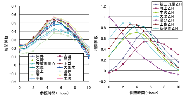
図－6 相関係数（左：水位変化－雨量、右：水位変化－水位変化）
