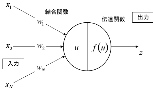
図-2 ANN構成素子の模式図
