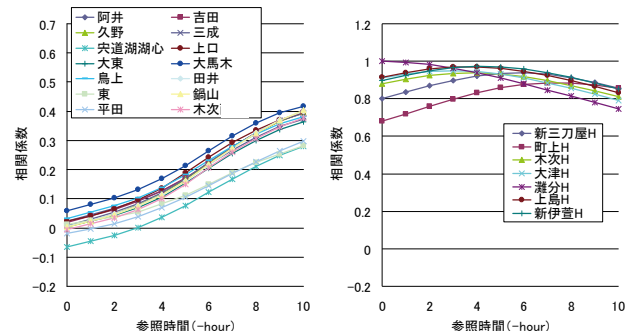
図－7 相関係数（左：水位－雨量、右：水位－水位）
