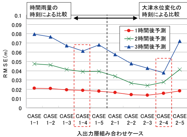
図－9 観測水位と予測水位の RMSE
