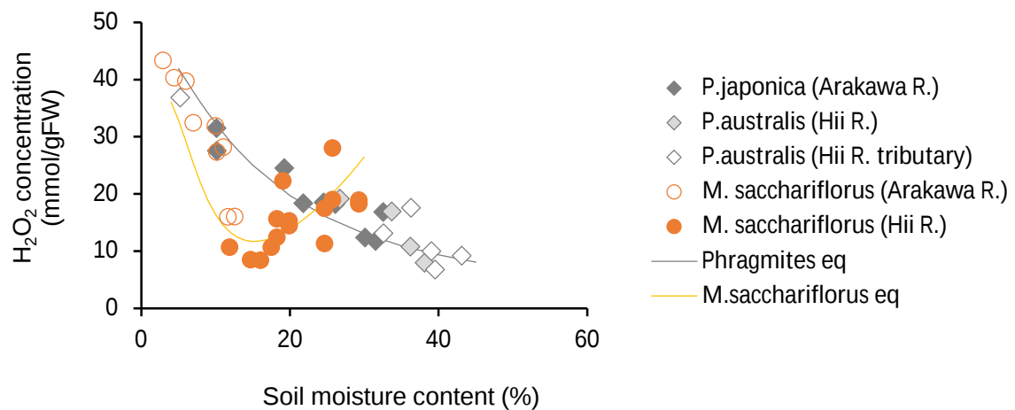
図4 草本類の ROS ( H_2O_2 濃度 ) と土壌水分の関係
