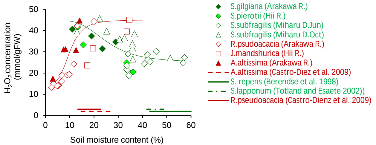
図3 木本類の ROS ( H_2O_2 濃度 ) と土壌水分の関係
