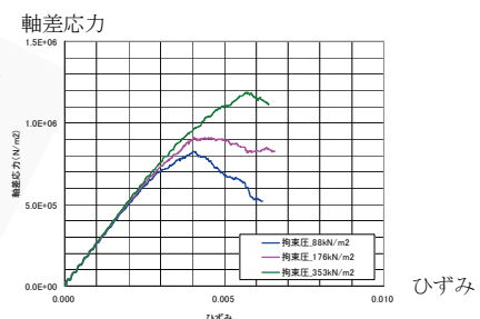
DEMによる大型室内実験のシミュレーション
