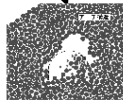
DEM モデル：球形粒子の集合で斜面をモデル化し、トンネルの崩壊をシミュレート
